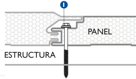
1 Tornillo con cabeza hexagonal de 1/4" x n"
